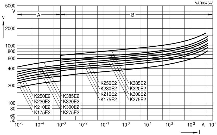
SIOV-SFS14K175E2 ... K385E2
